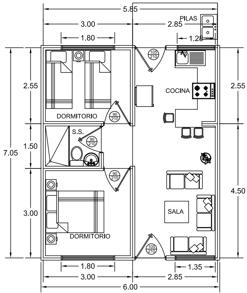
PLANTA DE DISTRIBUCION ARQUITECTONICA
