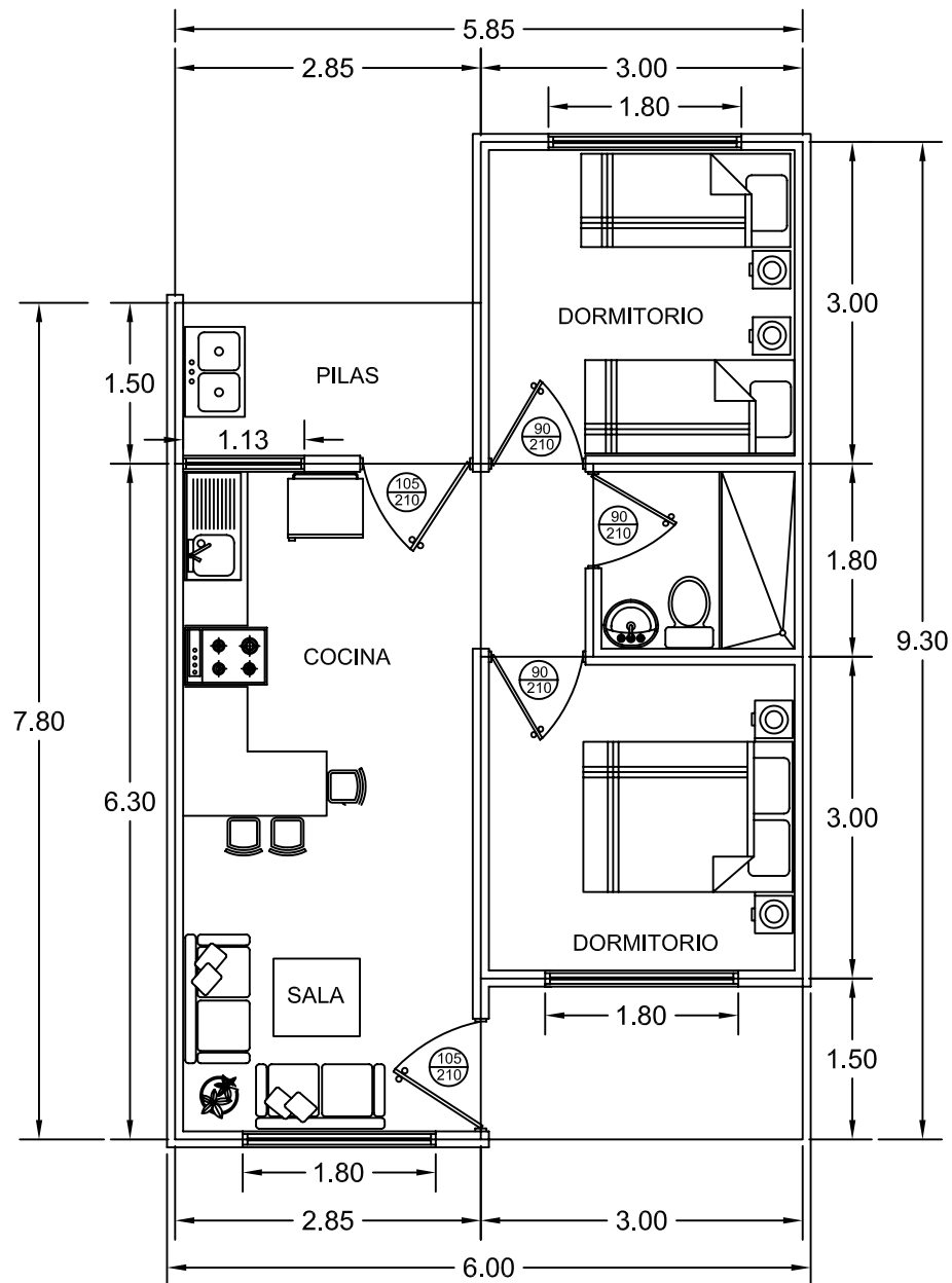
PLANTA DE DISTRIBUCION ARQUITECTONICA
