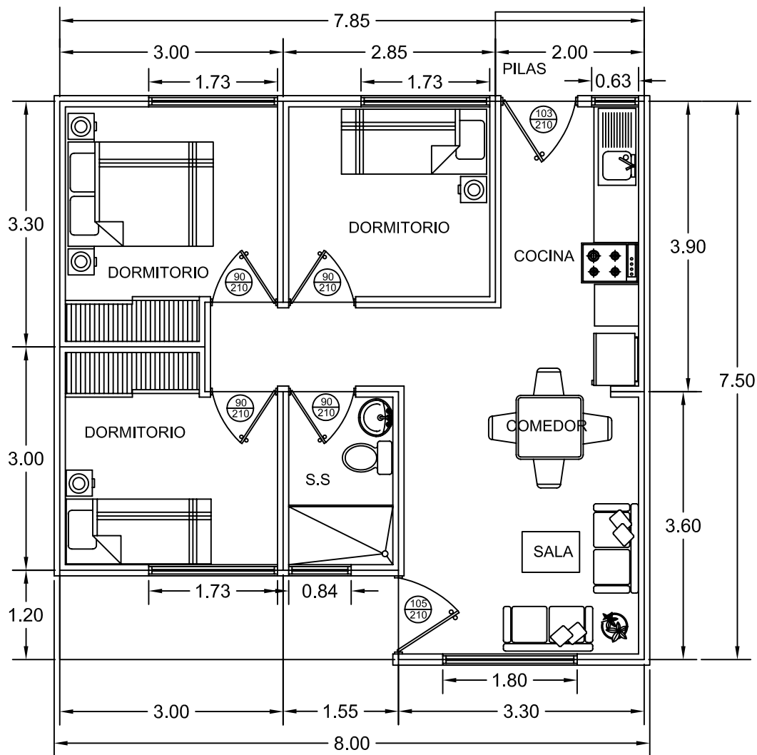
PLANTA DE DISTRIBUCION ARQUITECTONICA
