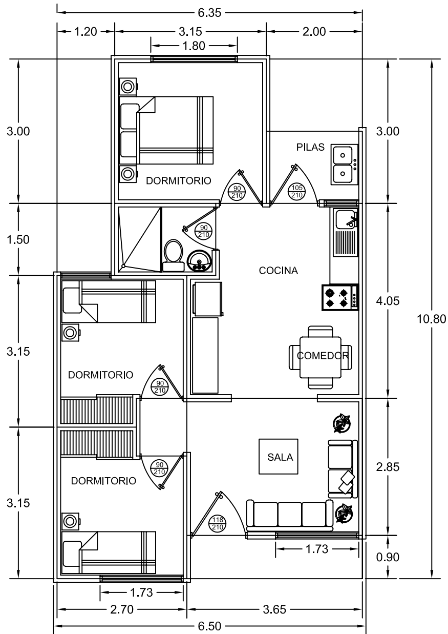
PLANTA DE DISTRIBUCION ARQUITECTONICA
