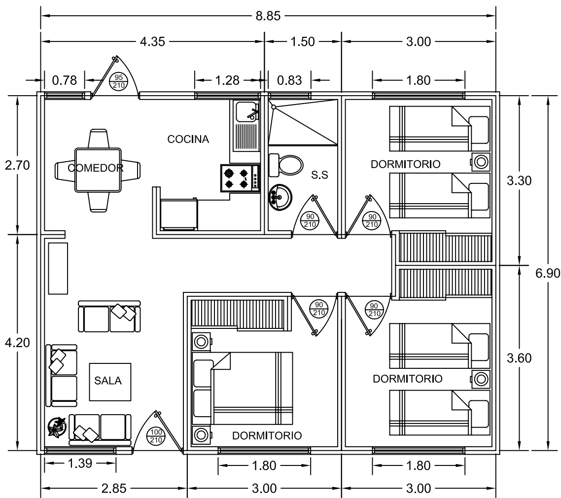
PLANTA DE DISTRIBUCION ARQUITECTONICA
