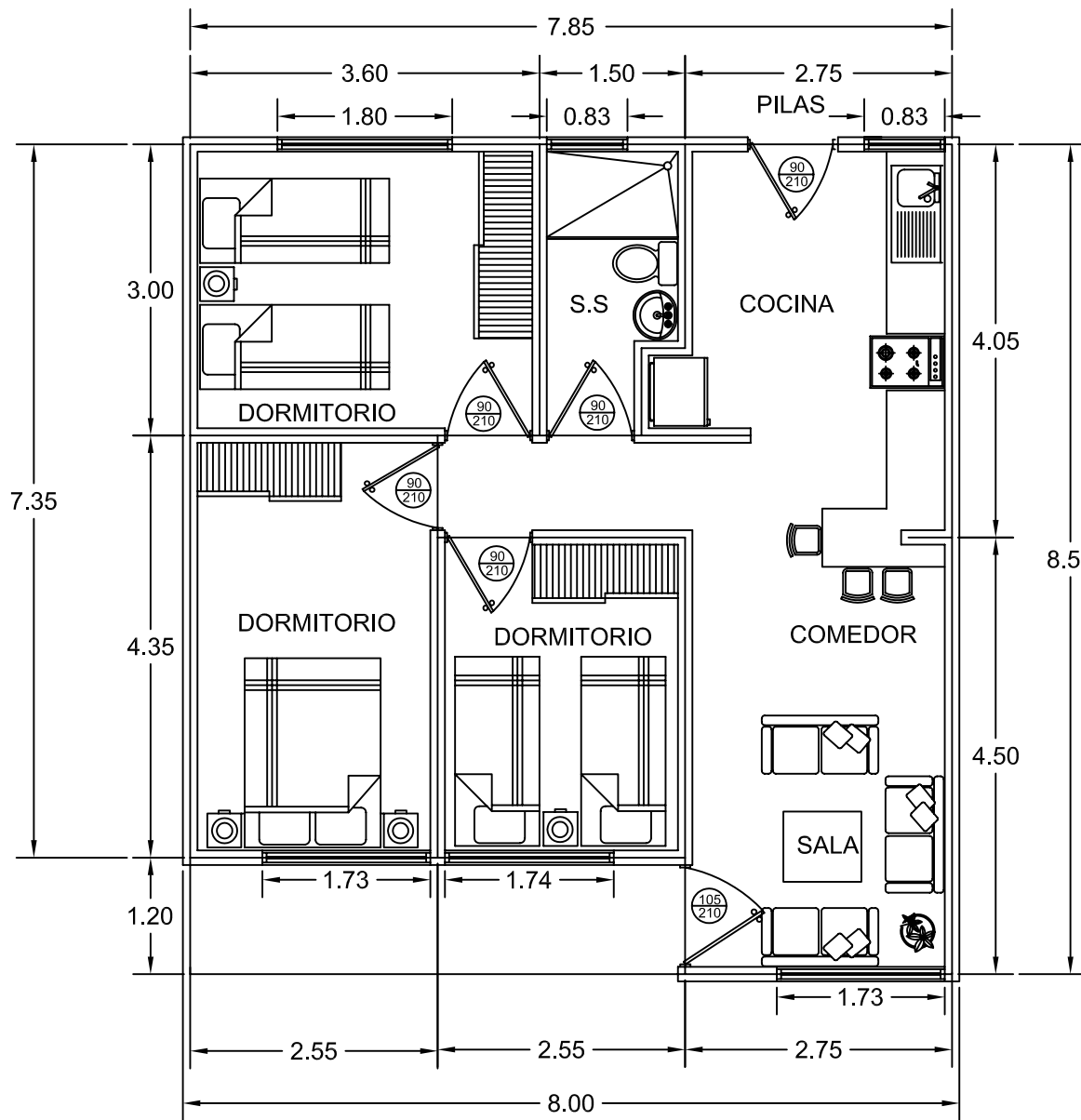
PLANTA DE DISTRIBUCION ARQUITECTONICA
