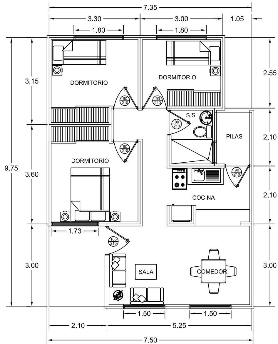
PLANTA DE DISTRIBUCION ARQUITECTONICA
