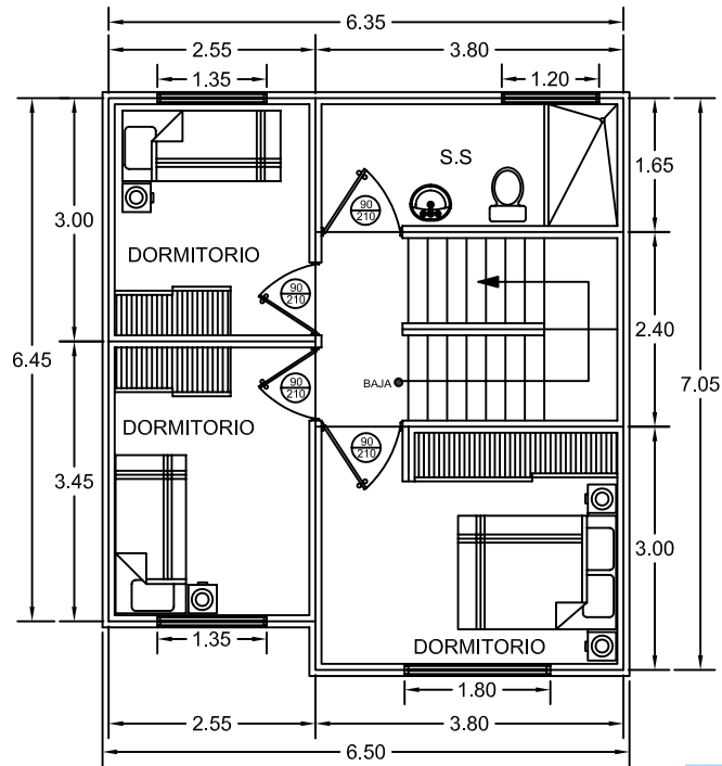
PLANTA DE DISTRIBUCION ARQUITECTONICA II NIVEL
