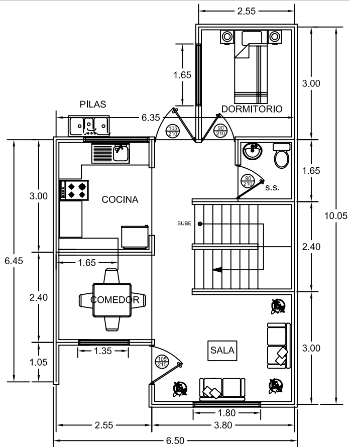
PLANTA DE DISTRIBUCION ARQUITECTONICA I NIVEL
